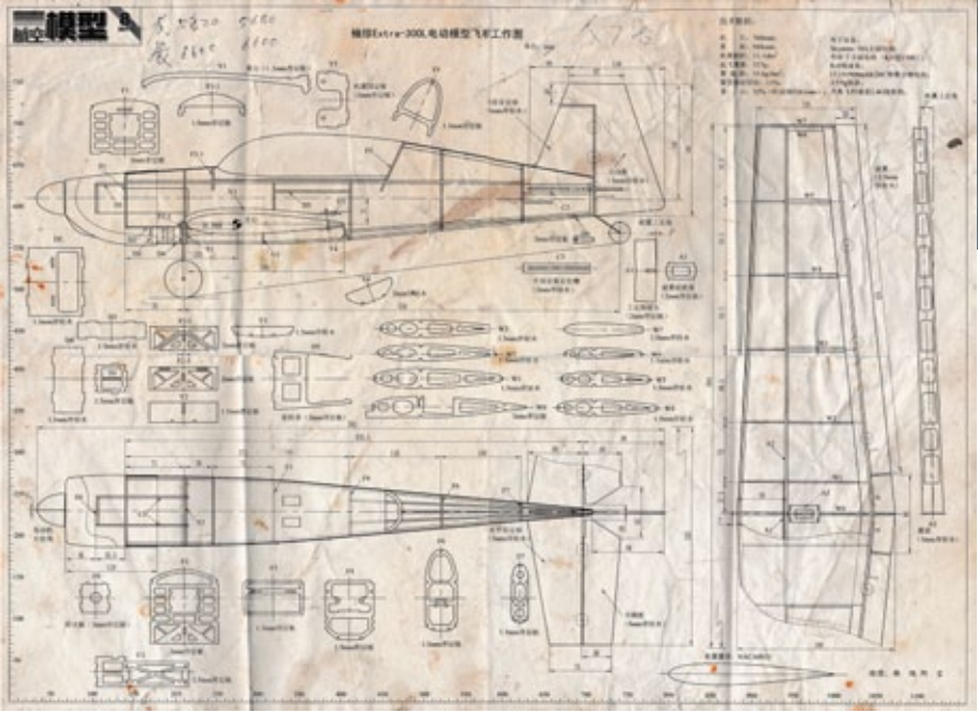
Bouwtekening van het vliegtuig van Jin Shaozhi.
