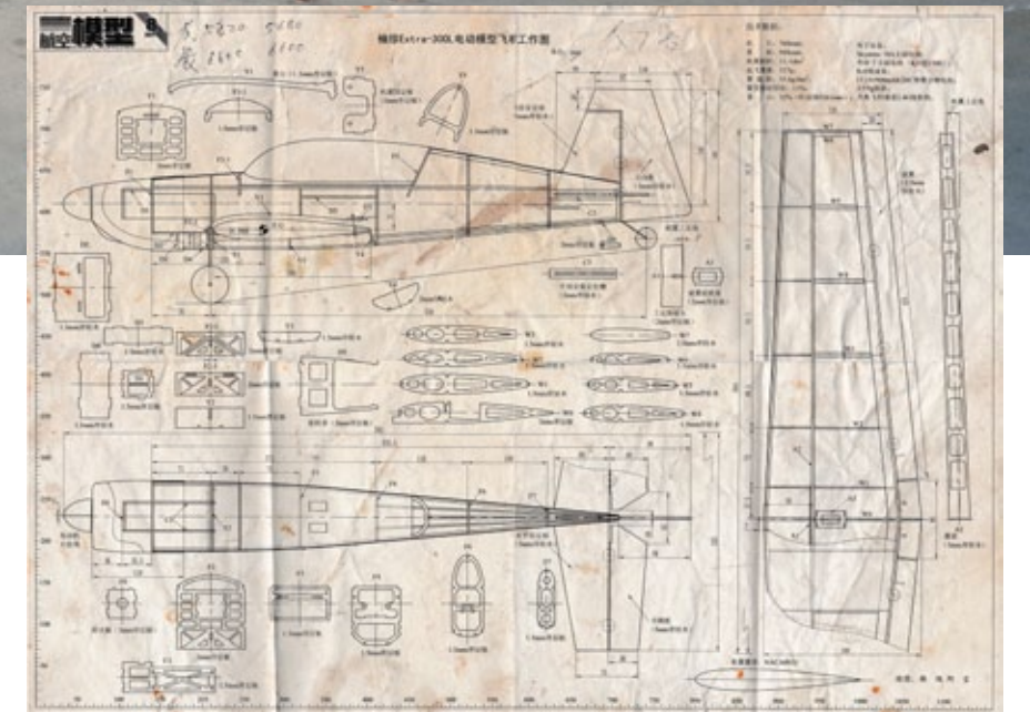
Bouwtekening van het vliegtuig van Jin Shaozhi.
